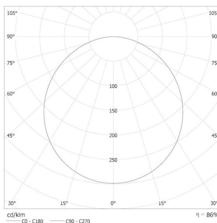
KANLUX S.A. (kat 37275) BLINGO NT 34W 6060 / Krzywa rozsyłu światła (biegunowo)
